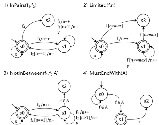
Fig. 3. Constraint Automata
