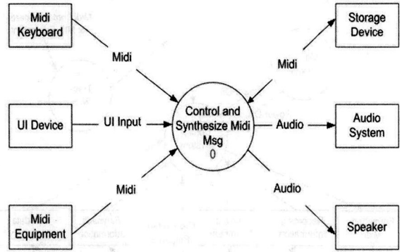
(그림 3) 뮤직 임베디드시스템의 컨텍스트 다이어그램
