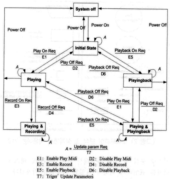
(그림 6) Control State Transition(CST) 다이어그램
