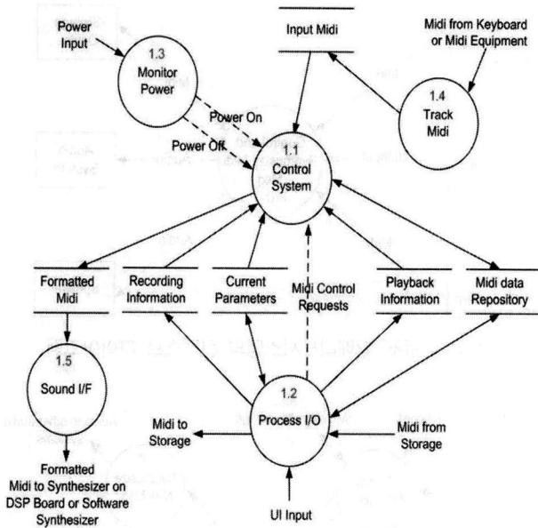
(그림 5) Control Midi Msg DFD
