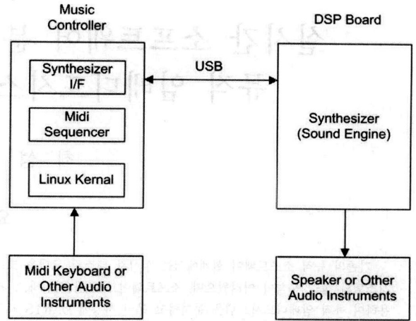
(그림 1) 뮤직 임베디드시스템의 구성
