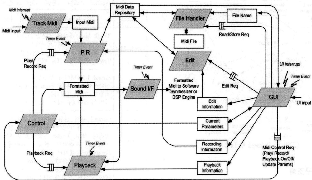
(그림 9) 태스크 아키텍처 다이어그램
