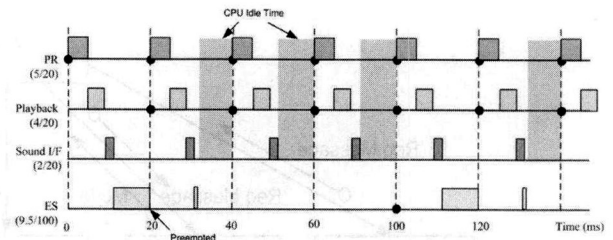
(그림 12) 태스크 실행 타이밍 차트
