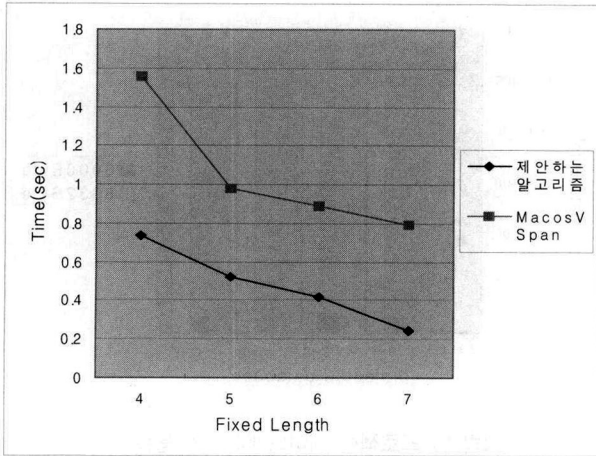
(그림 6) MacosVSpan과 제안하는 알고리즘의 검색성능 비교
