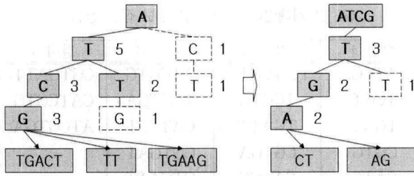
(그림 1) 고정길이 span method
