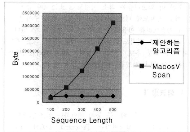
(그림 8) 두 알고리즘에 사용된 메모리량
