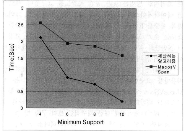
(그림 7) 최소지지도 변화에 따른 검색속도
