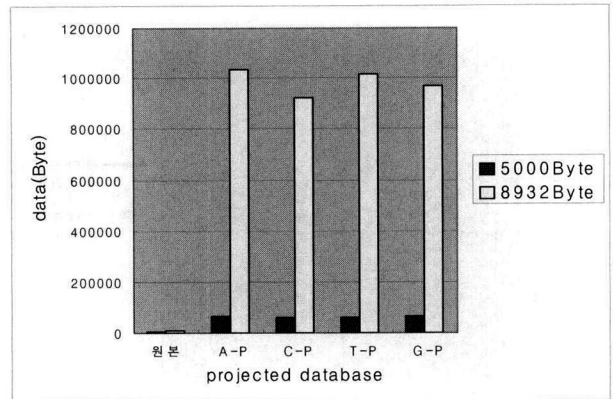
(그림 5) 프로젝션 데이터베이스의 용량비교
