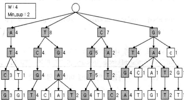
(그림 4) 고정길이 확장 트리 구축
