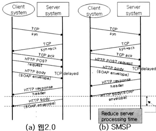
(그림 6) 웹 2.0과 SMSP의 이벤트 추적
