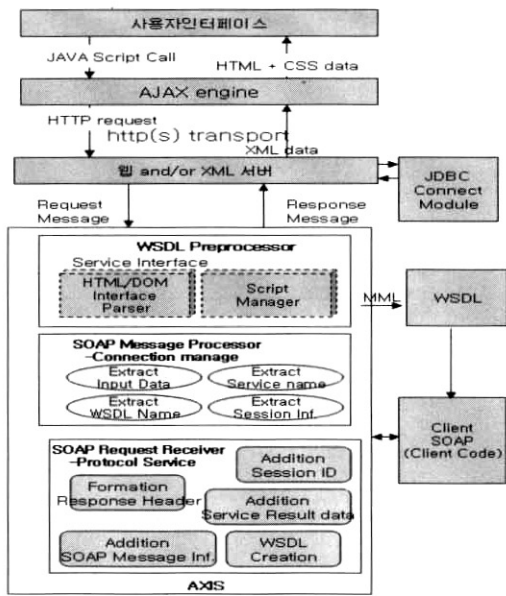
(그림 3) 실행된 SOAP Message Processor(SMSP) 구현
