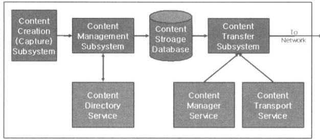
(그림 7) 콘텐츠 공유를 위한 IEEE1394 DMS 구성도
