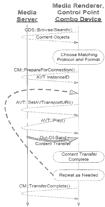
(그림 3) AV 콘텐츠 전송 절차
