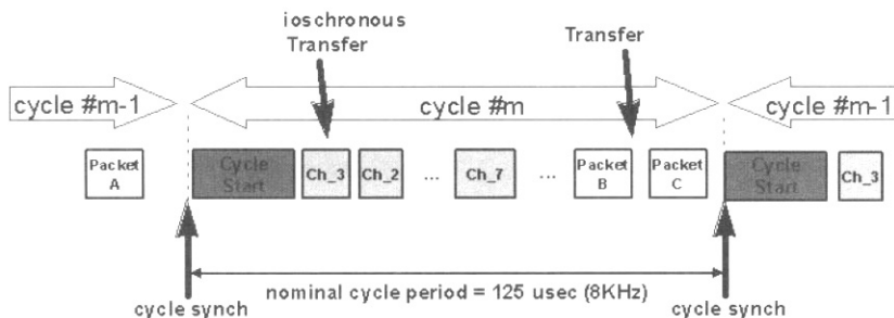
(그림 2) IEEE1394의 트랜잭션
