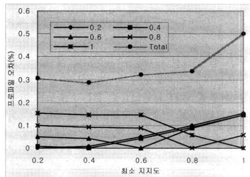
(그림 16) 최적 최소 지지도 탐색을 위한 프로파일의 상대 오차 비교
