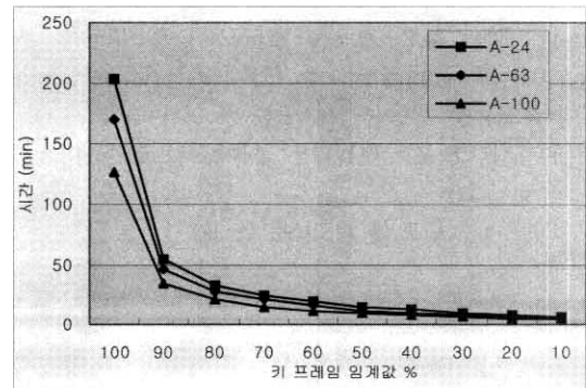
(그림 14) 키 프레임 압축을 사용에 따른 수행 시간 단축
