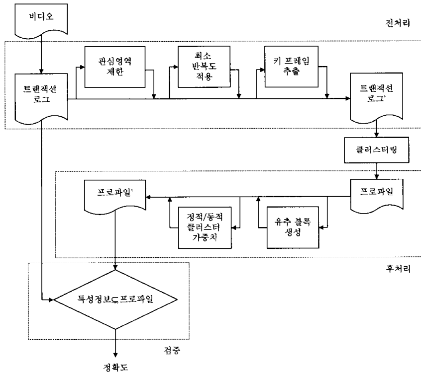
(그림 4) 비디오 데이터 집합의 특성정보 프로파일 생성 과정
