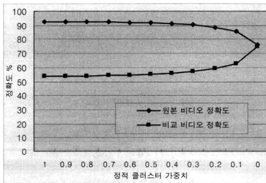
(그림 13) 클러스터 가중치 차별화에 따른 정확도의 변화
