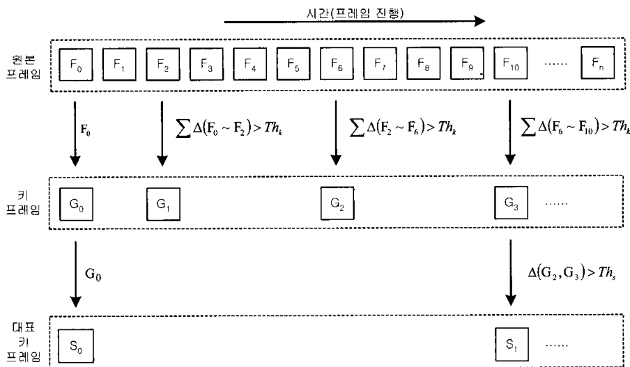
(그림 6) 키 프레임 추출 기법 적용 예제
