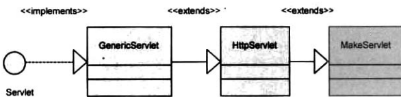
(그림 2) 서블릿 상속 관계
