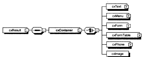
(그림 9) XML DTD 상충부
