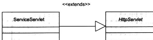
(그림 6) 서블릿 클래스
