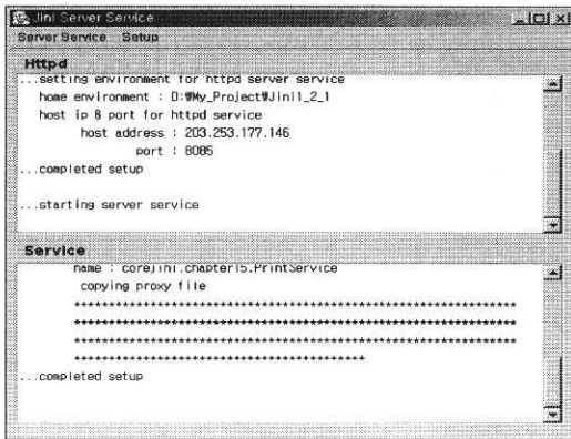
(b) 서버 서비스 실행
