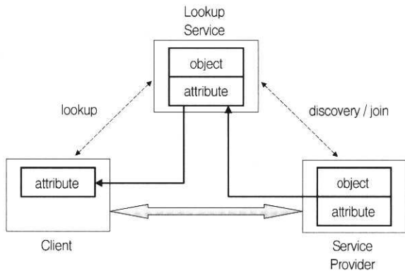
(그림 3) 지니 서비스 구조
