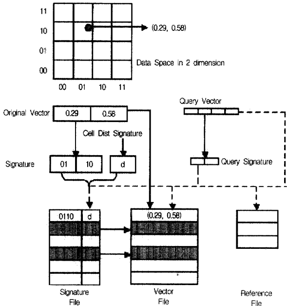
(그림 2) 셀기반 필터링 기법의 저장 및 검색
