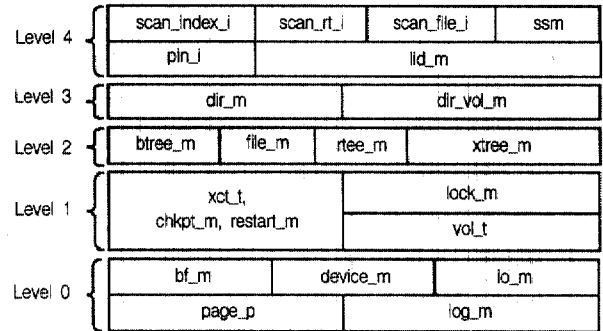
(그림 3) 확장된 SHORE 하부저장 시스템의 계층 구조
