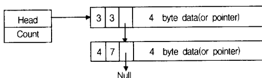
(그림 10) Delta queue 구조
