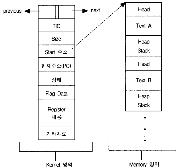
(그림 2) 다중 타스크를 지원하는 커널에서의 TCB 구조
