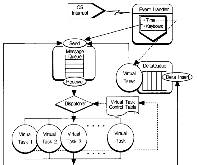
(그림 5) 추상 커널 계층 개념 구조도
