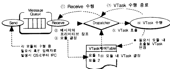
(그림 7) Dispatcher Running 과정
