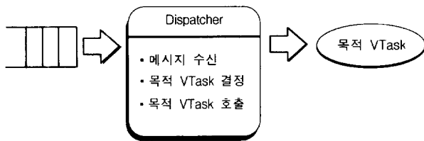
(그림 4) 추상 커널 계층 Dispatcher
