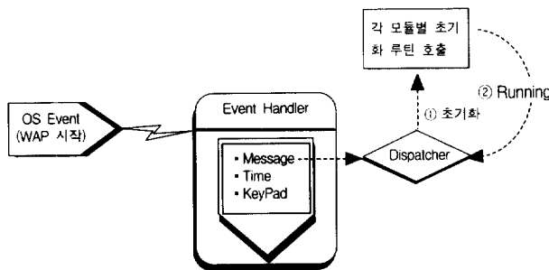
(그림 6) Dispatcher를 통한 모듈별 초기화
