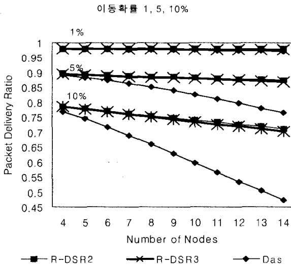
(그림 8) 메시지 전달률(이동확률 1,5,10%)
