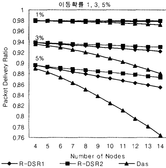
(그림 7) 메시지 전달률(이동확률 1,3,5%)
