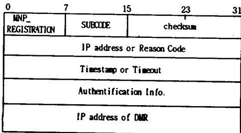
(그림 4) MH등록을 위한 MNP 패킷 (Fig. 4) MNP Packet for registration OF MH
