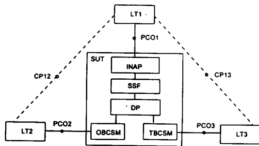
(그림 3) SSP 시험 형상 (Fig. 3) Test configuration for testing SSP
