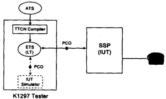
(그림 17) SSP 적합성 시험 환경 (Fig. 17) SSP conformance testing environment
