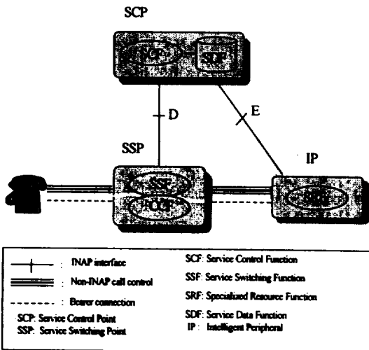
(그림 2) 차세대 지능망 구조 (Fig. 2) AIN architecture
