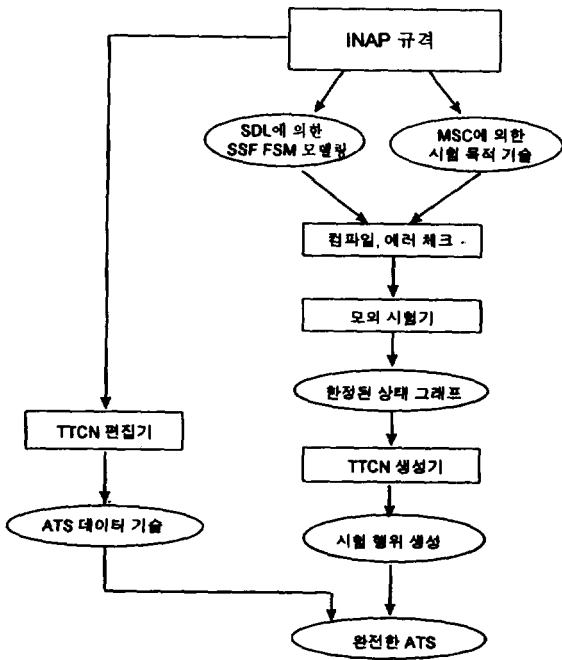
(그림 4) ATS 생성 절차
