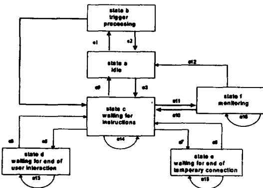
(그림 6) SSF FSM 상태 천이도 (Fig. 6) SSF FSM state diagram
