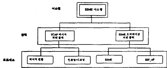
(그림 7) SSME 시스템 구조도 (Fig. 7) SSME system hierarchy diagram
