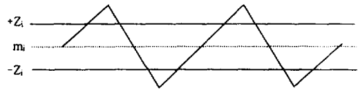
(그림 5) 위사 계산을 위한 영역 교차법 (Fig. 5) Zone-crossing method for weft calculation.
