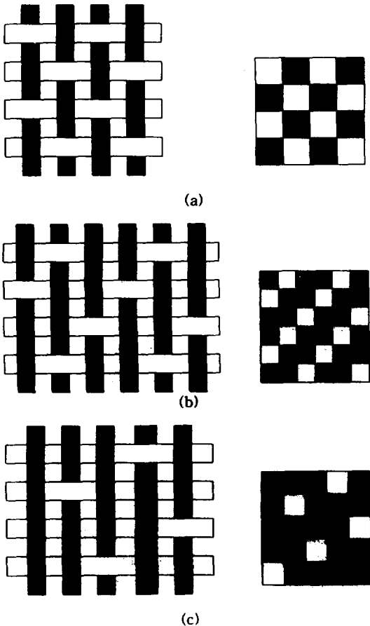
(그림 1) 3 원조직의 구조와 조직 (a) 평직 (b) 능직 (c) 주자직
