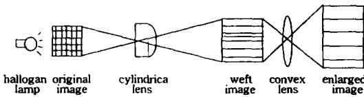
(그림 2) 밀도 측정 시스템 구성도 (Fig. 2) Configuration of density measurement system.
