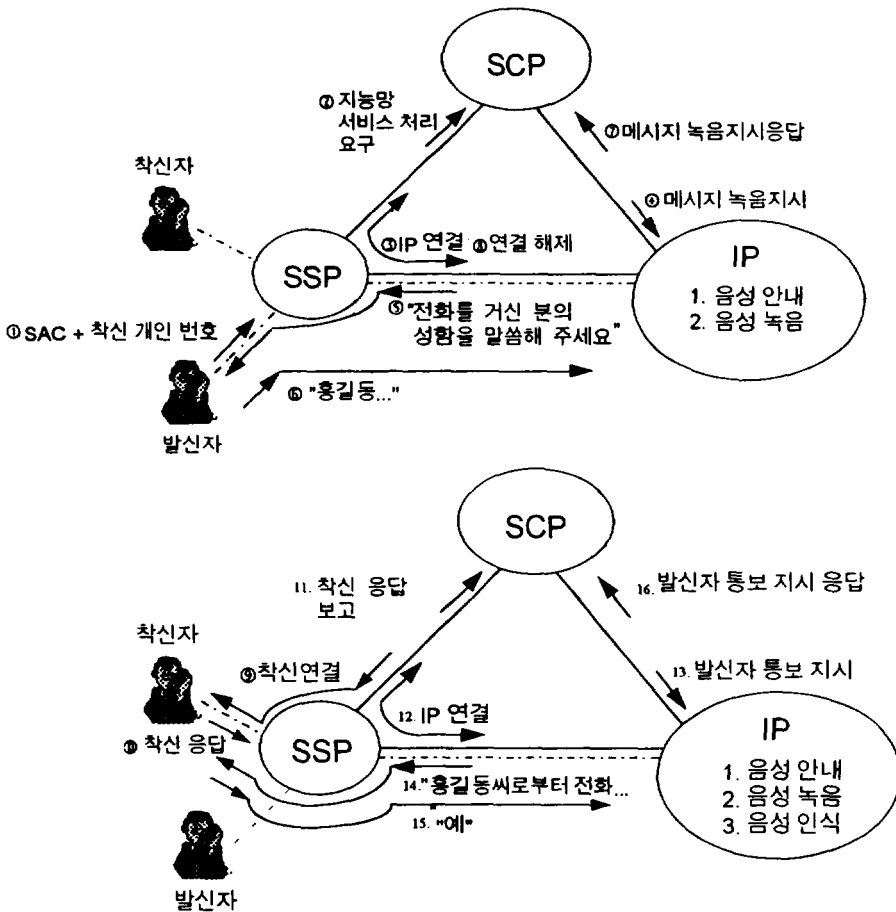
(그림 4) 음성 편집 기능의 예 : 발신자 통보 서비스 (Fig. 4) Example of Voice Synthesis : Announcement of Originating Party
