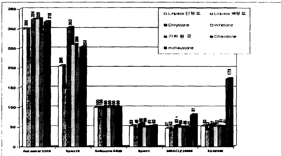
(그림 4) Chaustone과 다른 벤치마크들 실행 결과 (Fig. 4) The execution result of Chaustone and other benchmarks
