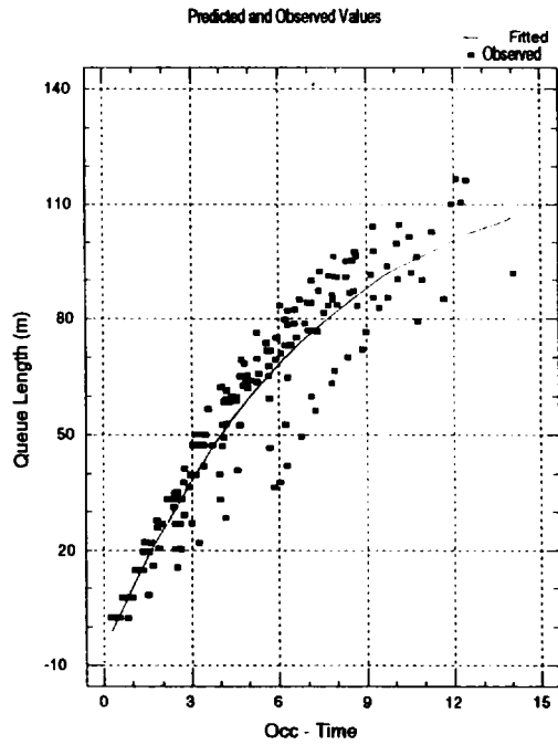
(그림 2-2.c) 10개주기 - 3차함수곡선 (Fig. 2-2.c) 10cycles - cubic function with quadratic terms
