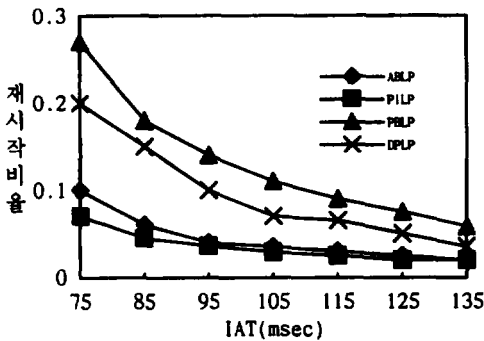
(그림 5) 잠금 프로토콜들의 IAT 변화에 따른 재시작 비율 (Fig. 5) Restart ratio to IAT locking protocols
