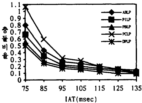
(그림 4) 잠금 프로토콜들의 IAT 변화에 따른 conflict-ratio 결과값
