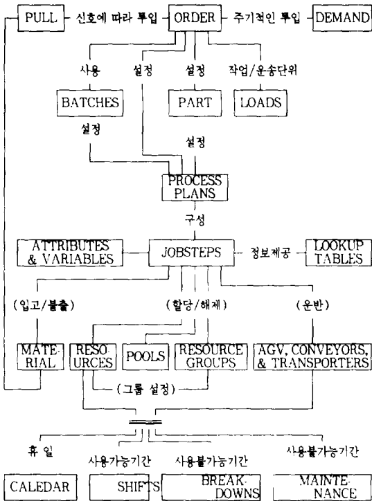
(그림 1) 시뮬레이션모델 요소 관계도
