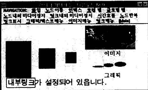
(그림 21) 그림 20상태에서 앵커영역을 클릭한 상태 (Fig. 21) State clicking anchor area in (Fig. 20) state
