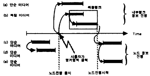
(그림 6) 노드 내에서의 중지/재시작 진행 (노드 정보 중지/재시작, 내부 링크의 정보 진행)
