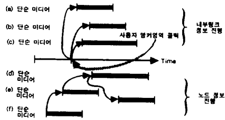
(그림 5) 노드 내에서의 동시 진행(노드 정보 진행, 내부 링크의 정보 진행)
