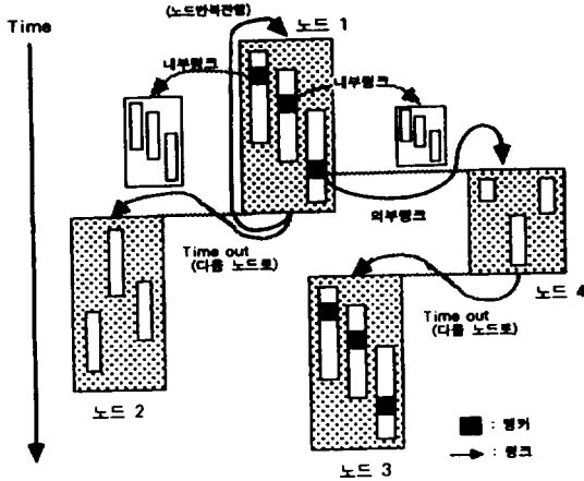
(그림 2) 동적 노드를 갖는 제한된 하이퍼미디어의 노드 관계 (Fig. 2) Node relations of the proposed hypermedia with dynamic nodes
