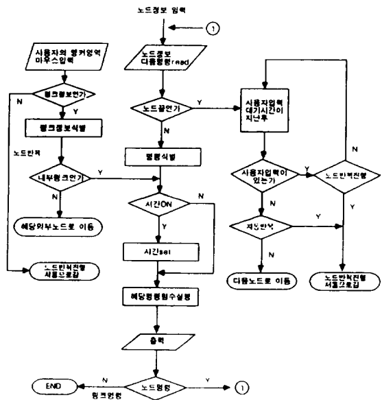
(그림 16) 동적 노드 명령 처리기의 내부 처리 과정 (Fig. 16) Internal process of dynamic node instruction processor
