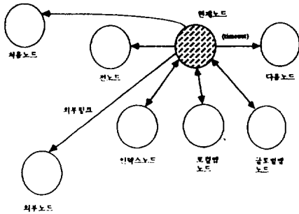
(그림 15) 현재노드와 관련된 노드들과의 관계 (Fig. 15) Relation between current node and associated nodes
