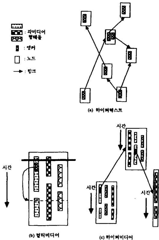
(그림 1) 하이퍼텍스트, 멀티미디어와 하이퍼미디어 (Fig. 1) Hypertext, multimedia and hypermedia
