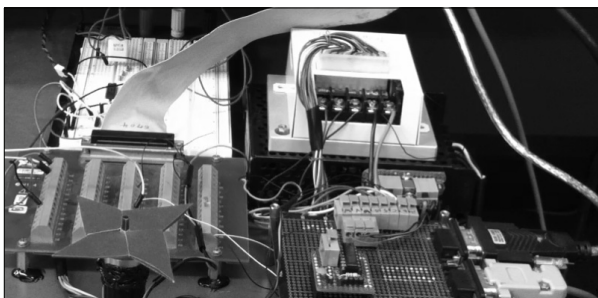
Fig. 3. Actual configuration of the BLDC motor controller test
