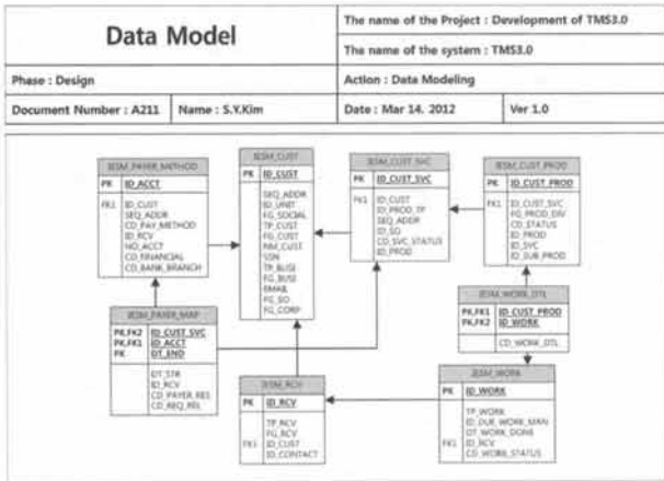
Fig. 9. Data Model
