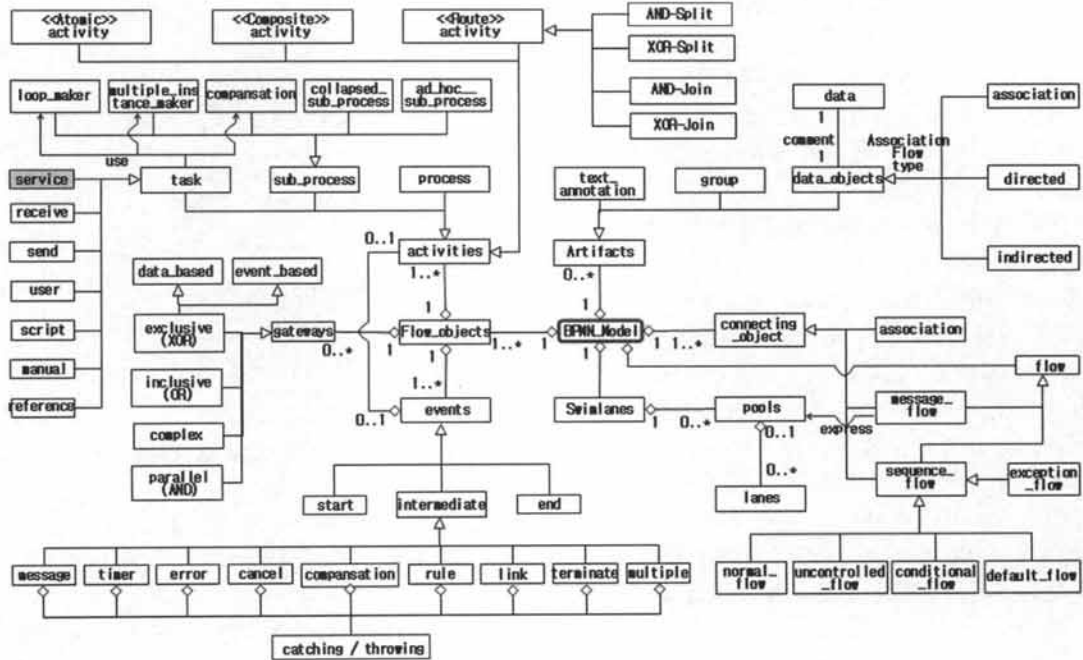
Fig. 4. BPMN metamodel
