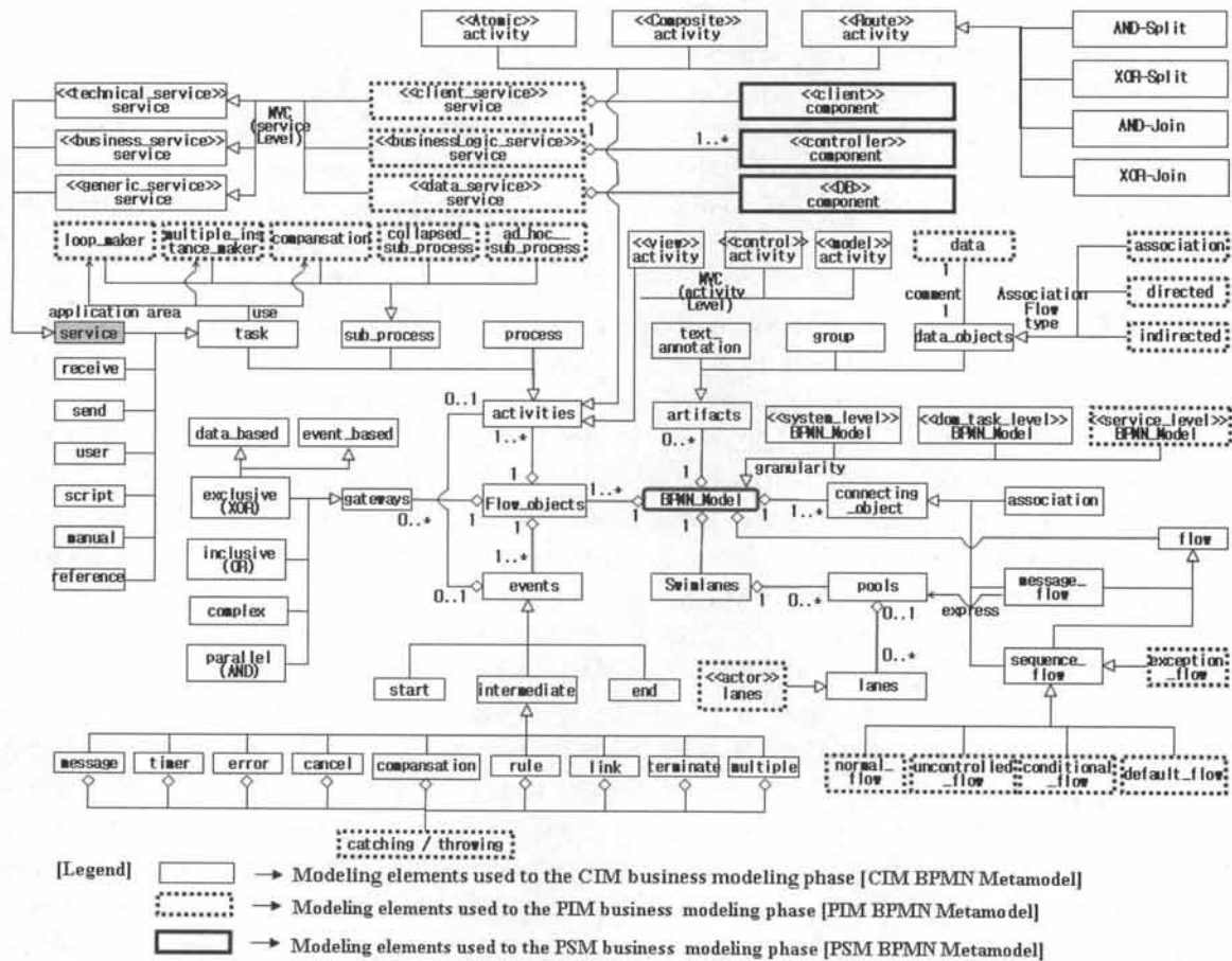
Fig. 6. XL-BPMN metamodel
