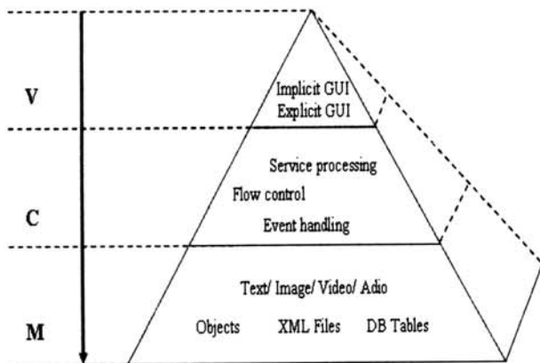
(그림 4) MVC view의 추상적 피라미드 구조
