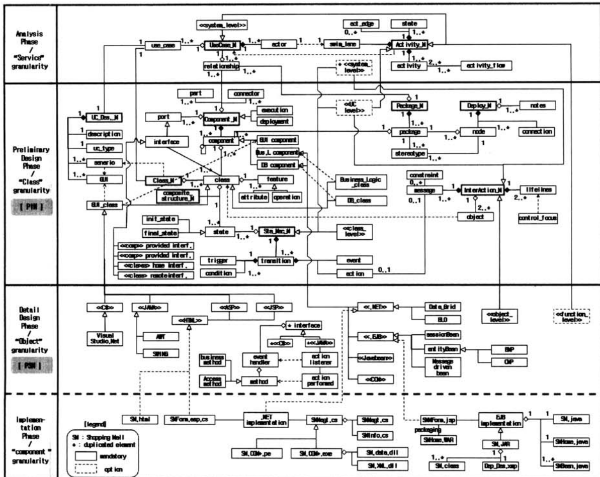
(그림 7) Process view 기반 계층적 통합 메타모델
