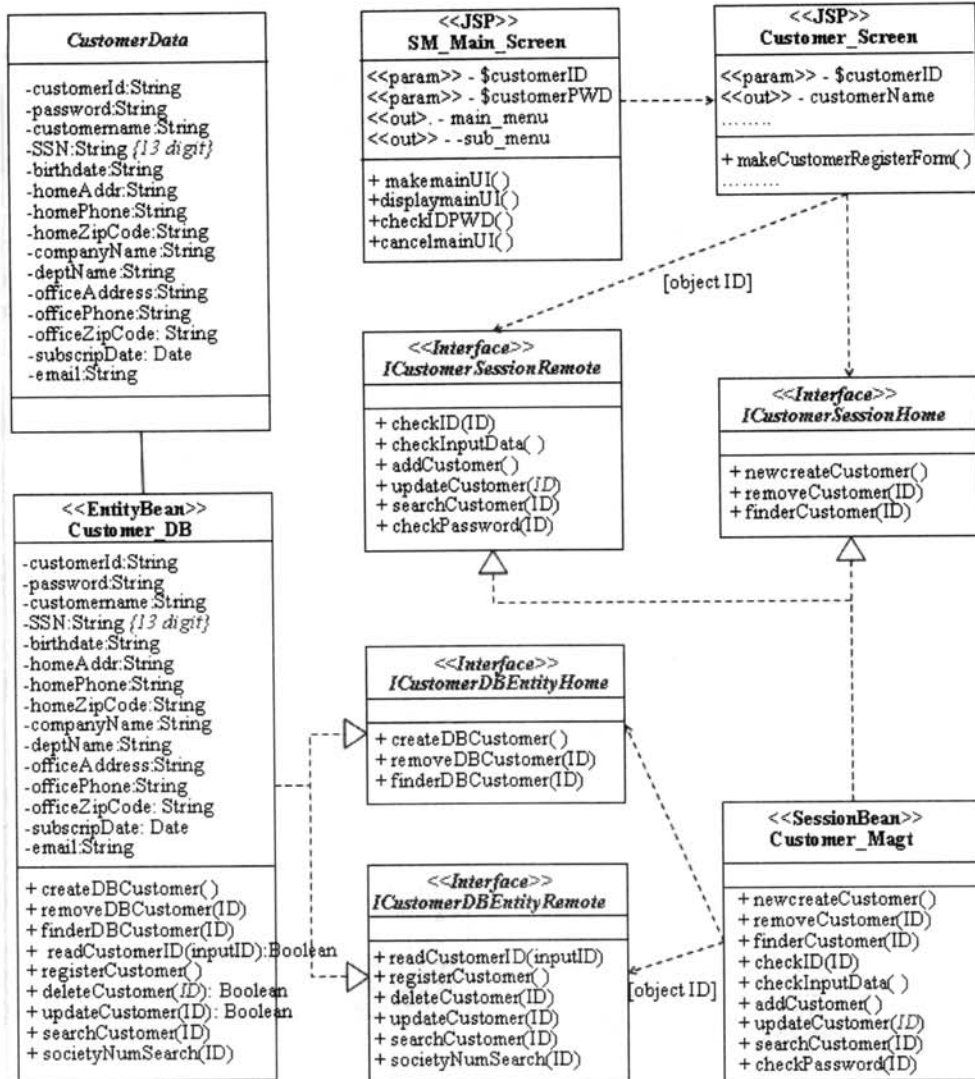
(그림 11) PSM Class model
