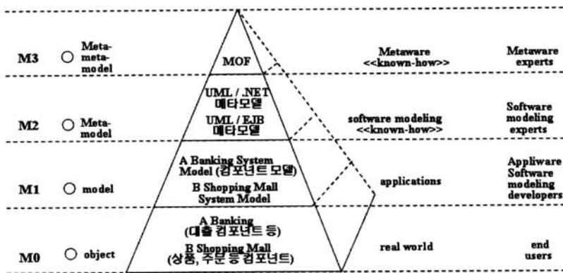
(그림 6) meta-architecture view 기반 계층적 메타모델
