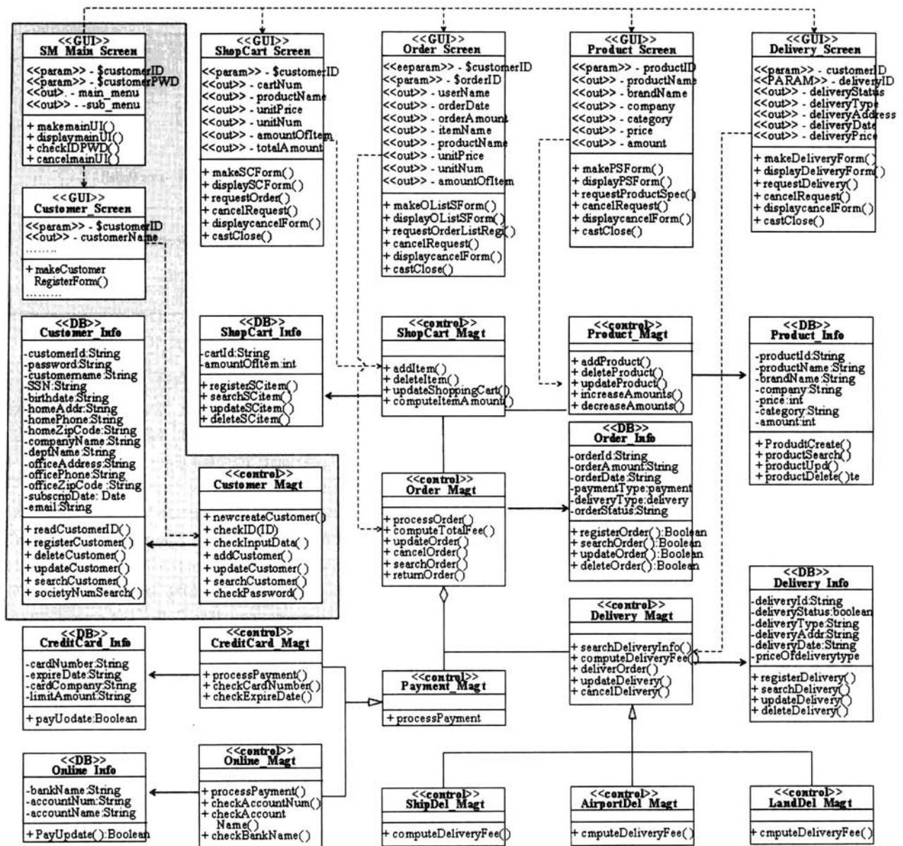
(그림 9) PIM Class model
