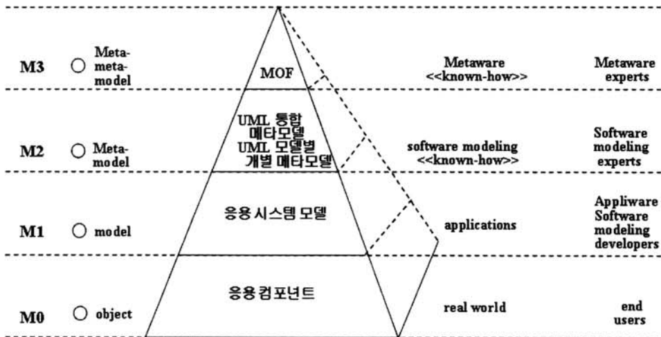
(그림 2) Meta-architecture view의 메타 피라미드 구조
