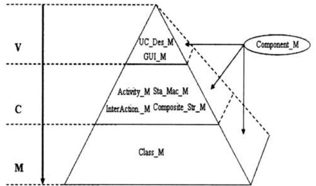
(그림 5) MVC view의 상세적 피라미드 구조
