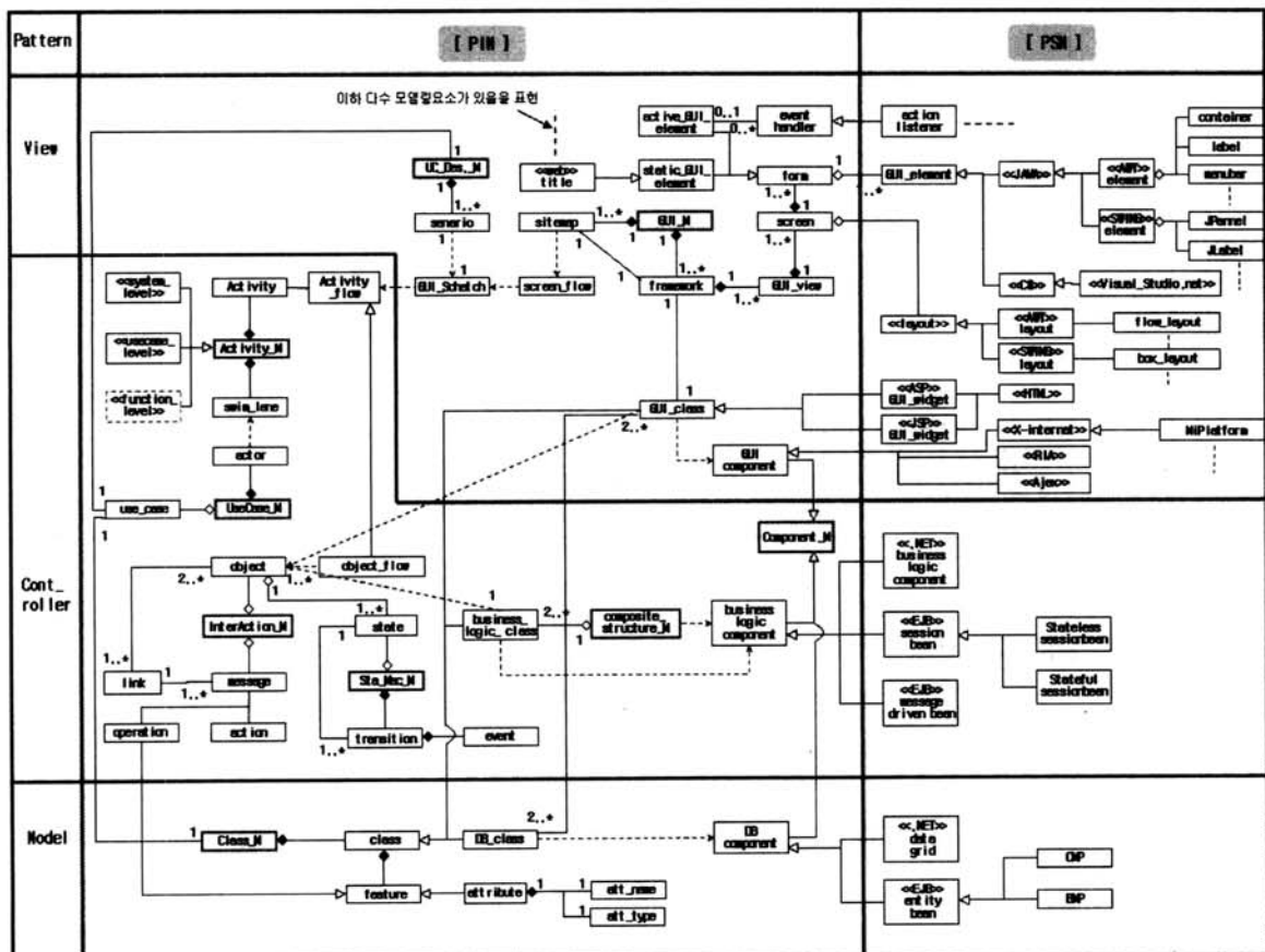
(그림 8) MVC view 기반 계층적 통합 메타모델
