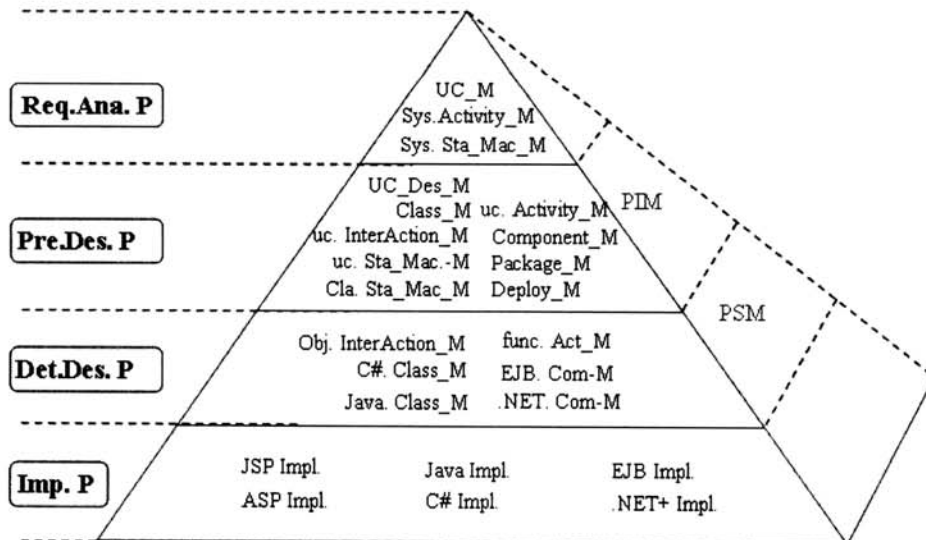
(그림 3) Process view의 피라미드 구조
