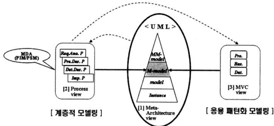
(그림 1) 2+1 view meta-architecture 모델
