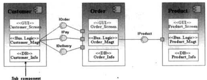
(그림 10) PIM Component model
