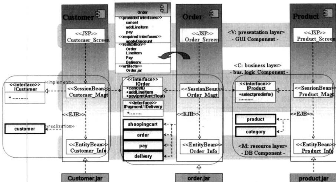
(그림 12) PSM Component model
