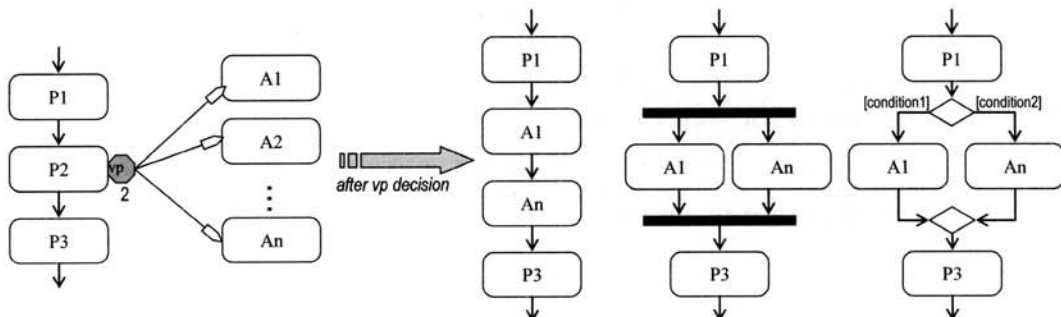
(그림 7) 둘 이상의 가변치가 선택될 수 있는 대체가능 후보선택 가변성
