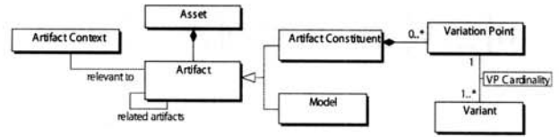
(그림 2) 소프트웨어 프로덕트 라인 자산 메타모델
