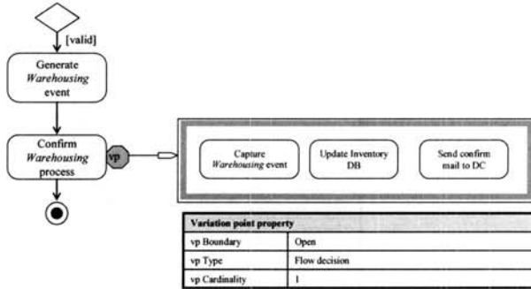
(그림 12) 흐름 결정 가변성을 가진 BPFM 예
