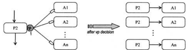
(그림 6) 하나의 가변치가 선택될 수 있는 대체가능 후보 선택 가변성
