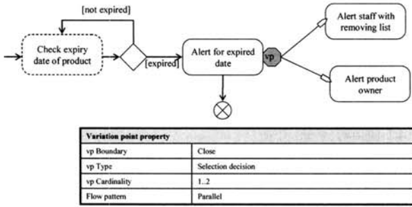
(그림 8) 대체가능 후보 선택 가변성을 가진 BPFM 예
