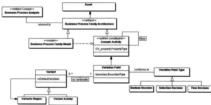
(그림 3) BPFM 메타모델
