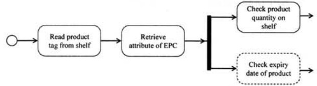
(그림 5) 유효기간 검사 액티비티 (Check expiry data of product) 가 선택성 속성 가변성으로 표현된 BPFM 예
