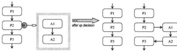
(그림 9) 확장 흐름 선택 가변성
