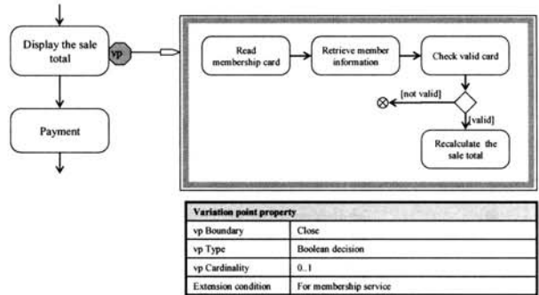
(그림 10) 확장 흐름 선택 가변성을 가진 BPFM 예
