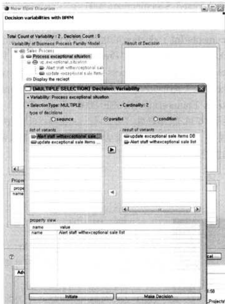
(그림 15) BPFM의 가변성 결정 사용자 인터페이스
