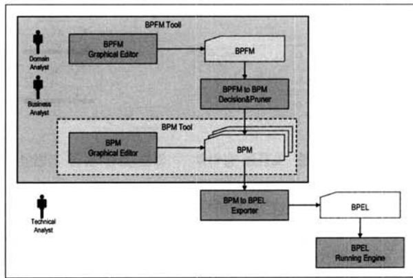
(그림 13) BPFM 기반 BPM 자동생성 도구 범위 및 주 기능 컴포넌트
