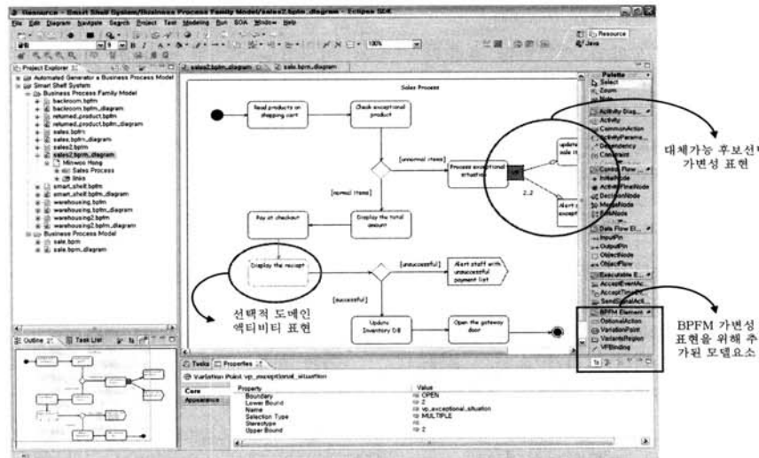
(그림 14) BPFM 개발을 위한 사용자 인터페이스
