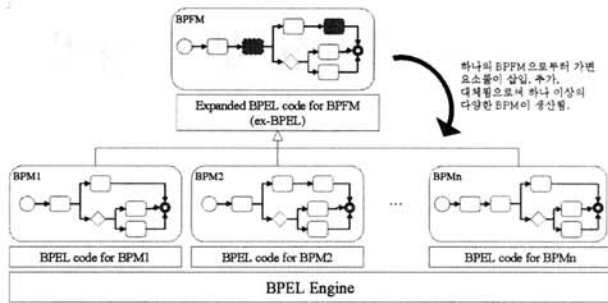
(그림 1) 하나의 BPFM로부터 유도되는 하나 이상의 BPM - BPFM 에서 회색 표시된 부분이 가변 될 수 있는 부분임을 나타냄
