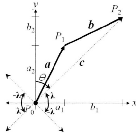
(그림 7) 두 벡터합
