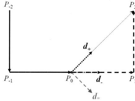
(그림 9) 단순 벡터합에 의한 평균 이동방향
