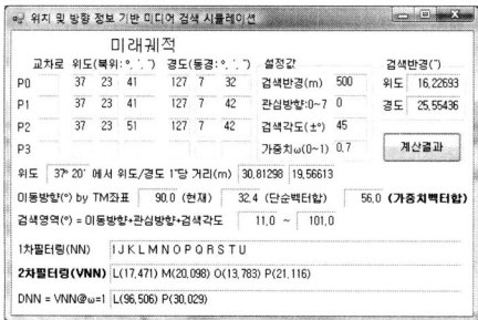
(그림 13) 검색 시뮬레이션
