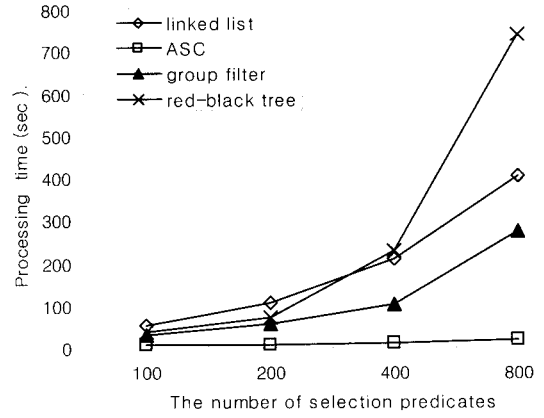
(b) 조건형태 : R.a \geq C_1 and R.a \leq C_2
