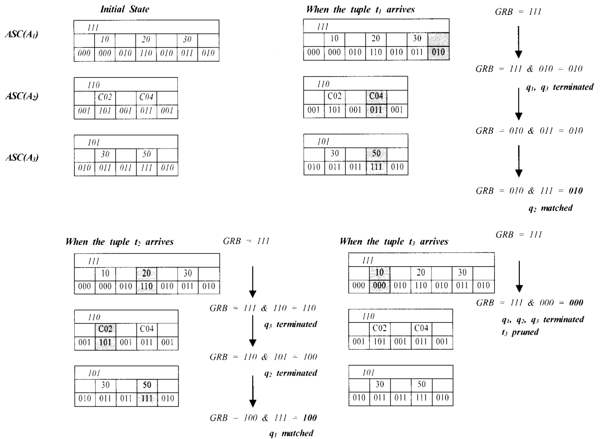
(그림 2) 속성 선택체를 이용한 데이터 스트림에 대한 다중 연속 질의 수행 예
