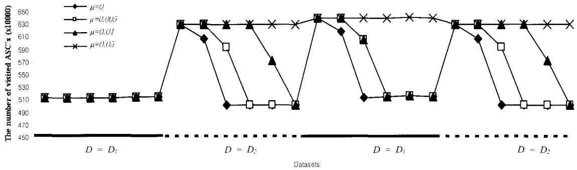
(그림 9) 재정렬 임계치 \mu 값에 따른 적응적 속성 선택체 처리 순서 재정렬 효과
