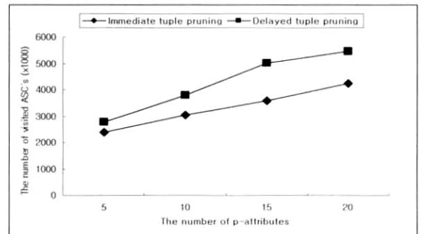
(그림 8) 튜플 제거 효과
