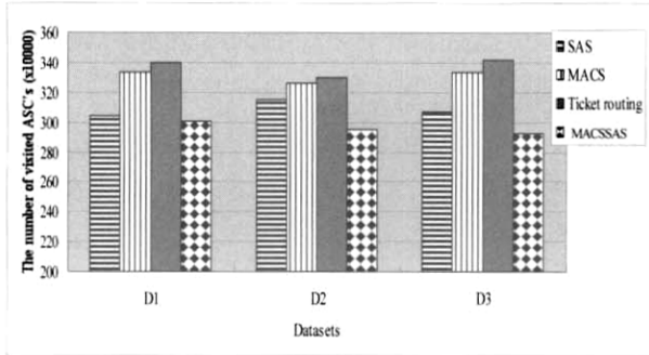
(a) 제안된 기법들과 티켓라우팅과의 비교
