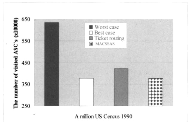
(그림 7) 실제 데이터집합을 대상으로 한 질의성능 비교
