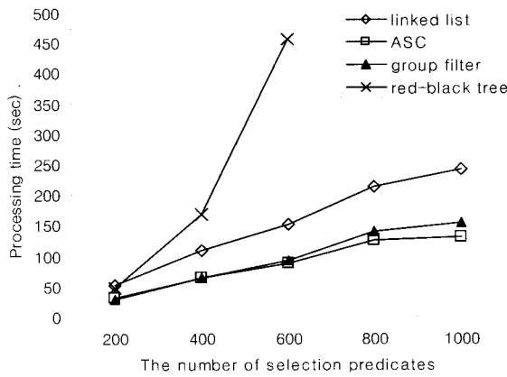
(a) 조건형태 : R.a \geq C
