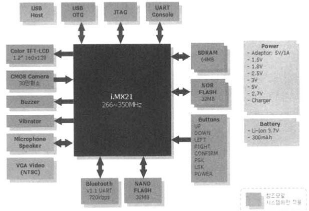
(그림 3) i.MX21 개발보드 및 WPS의 블록 다이어그램
