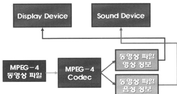
(그림 1) MPEG-4 동영상 플레이어의 전체적인 구조
