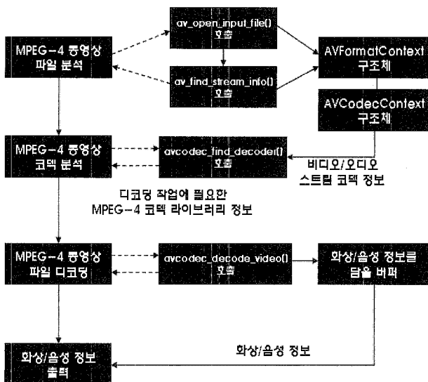
(그림 4) MPEG-4 동영상 플레이어의 전반적인 실행 과정
