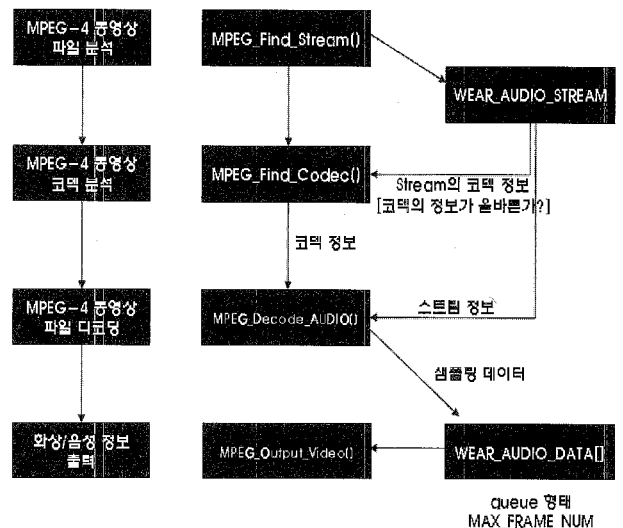
(그림 9) MPEG-4 동영상 플레이어의 오디오 출력 부분 구현
