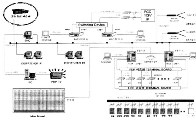
(그림 2) 전력감시제어설비의 시스템 구성도
