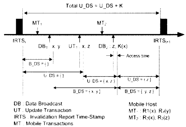
(그림 3) 서버 알고리즘의 예
