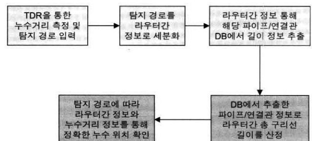
(그림 6) 이상위치 산출 알고리즘
