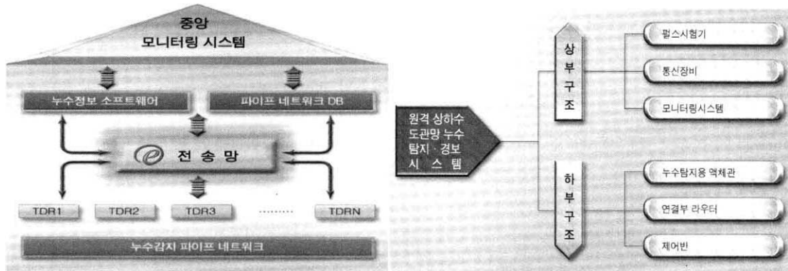
(그림 3) 중앙 모니터링 시스템 구성도와 구조도
