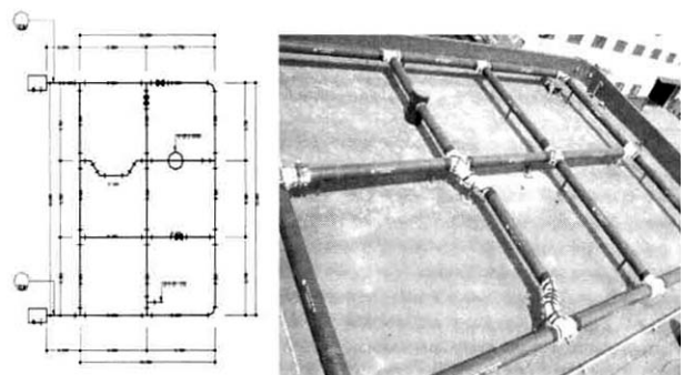
(그림 9) 파이로트 시스템 설계도와 구축한 파이로트 시스템
