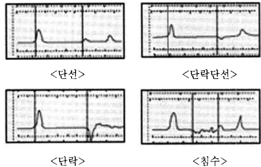
(그림 2) TDR 반사 파형 비교
