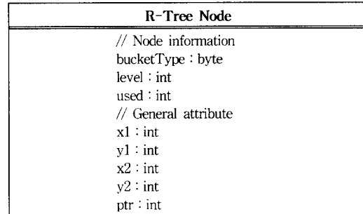
(그림 5) R-Tree 노드 클래스
