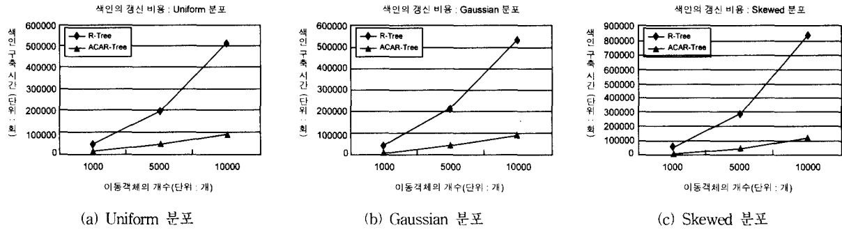
(그림 9) 데이터 분포별 색인의 갱신 성능 비교
