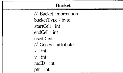
(그림 4) Bucket 클래스
