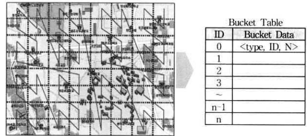
(그림 2) Z-Ordering 과정과 Bucket Table 구조
