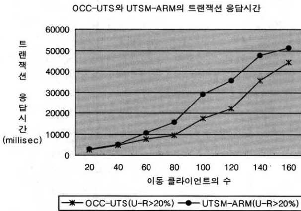
(그림 5-9) 이동 클라이언트수에 따른 트랜잭션 응답시간 (U-R = 20%)
