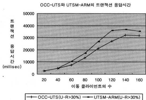
(그림 5-10) 이동 클라이언트수에 따른 트랜잭션 응답시간 (U-R = 30%)
