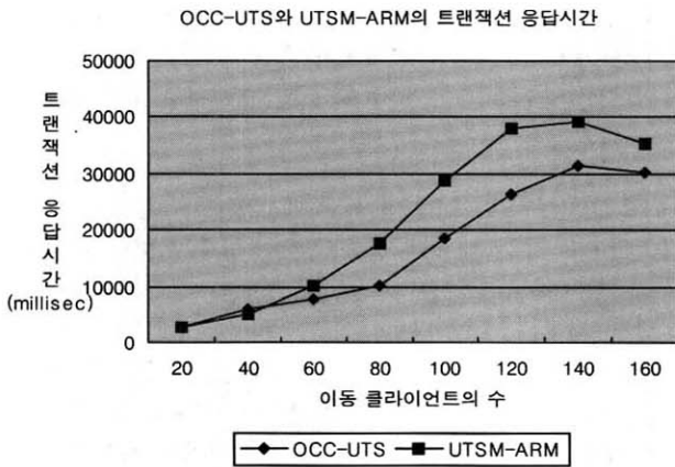
(그림 5-7) 이동 클라이언트수에 따른 트랜잭션 응답시간 (U=R)
