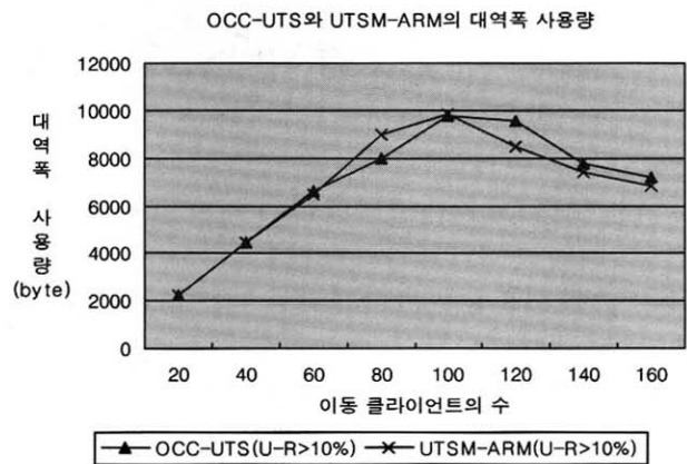
(그림 5-4) 이동 클라이언트수에 따른 메시지(Uplink)량 (U-R = 10%)
