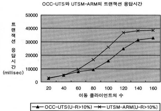
(그림 5-8) 이동 클라이언트수에 따른 트랜잭션 응답시간 (U-R=10%)
