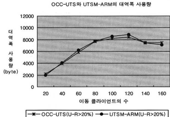
(그림 5-6) 이동 클라이언트수에 따른 메시지(Uplink)량 (U-R = 30%)
