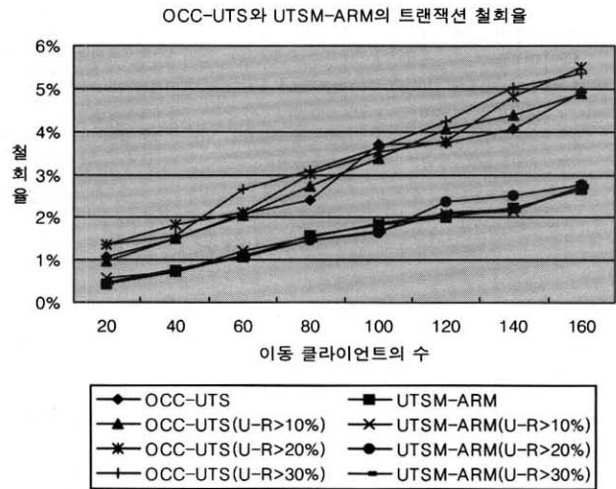
(그림 5-1) 이동 클라이언트 수에 따른 이동 트랜잭션의 철회율
