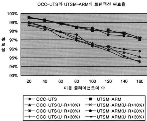
(그림 5-2) 이동 클라이언트 수에 따른 이동 트랜잭션의 완료율
