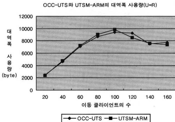
(그림 5-3) 이동 클라이언트수에 따른 메시지(Uplink)량 (U=R)
