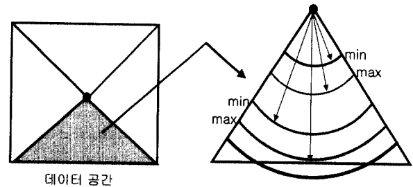
(그림 2.2) PdR-트리의 데이터 페이지 분할 방법
