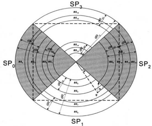
(그림 3.4) BS_i 까지의 최소거리 : 경우 3
