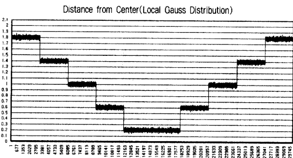
(그림 4.4) 지역 가우스 분포(Local Gauss Distribution)
