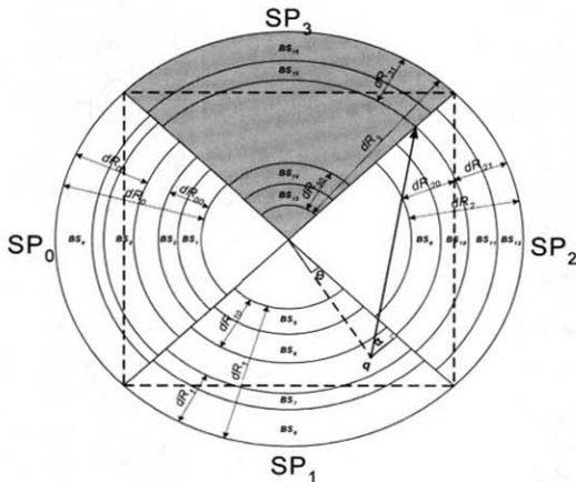
(그림 3.3) BS_i 까지의 최소 거리 : 경우 2
