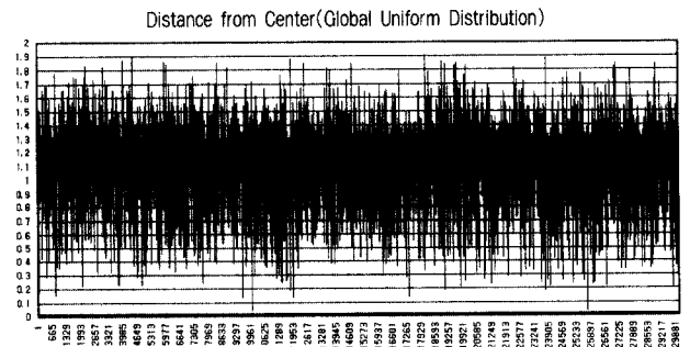
(그림 4.1) 전역 균등 분포(Global Uniform Distribution)
