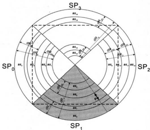
(그림 3.2) BS_i 까지의 최소 거리 : 경우 1
