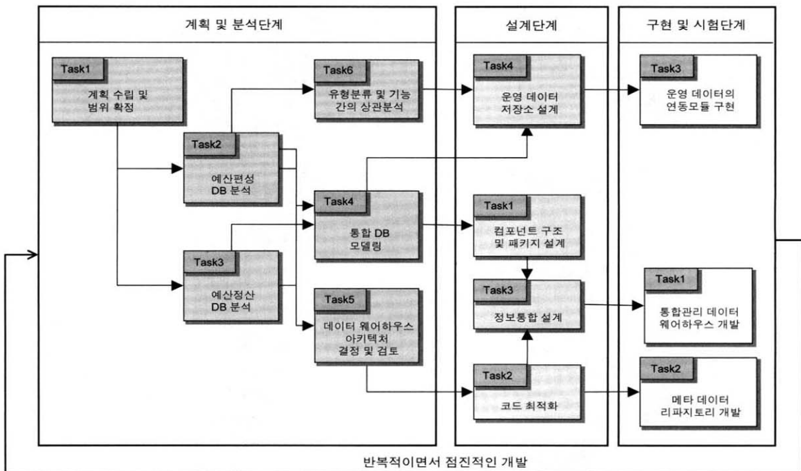
(그림 3) 엔터프라이즈 환경의 연구비 통합관리 데이터 웨어하우스 개발 프로세스
