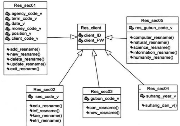
(그림 5) 예산편성 클래스 다이어그램
