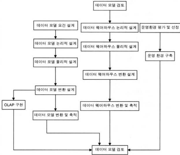
(그림 2) IBM의 데이터 웨어하우스 개발 프로세스
