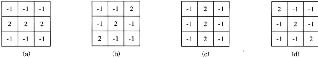
(그림 2) (a) 0° 방향 (b) 45° 방향 (c) 90° 방향 및 (d) 135° 방향의 라인 연산자
