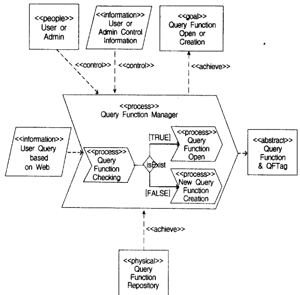
(그림 8) 질의 함수 관리기의 프로세스 다이어그램
