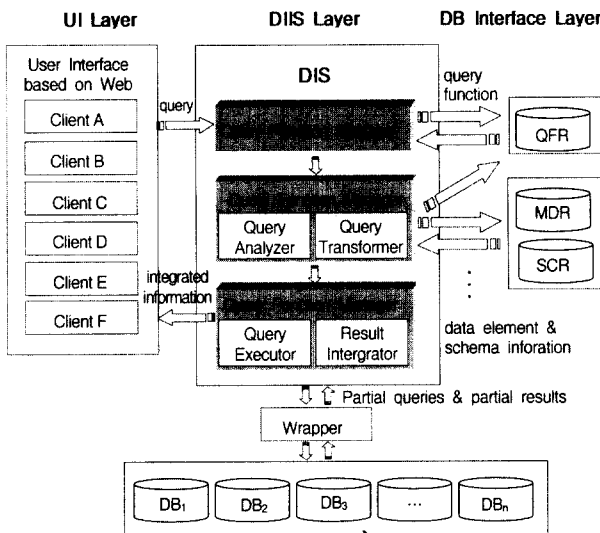
(그림 4) MDR 기반의 분산 정보 통합 시스템의 3계층 아키텍처
