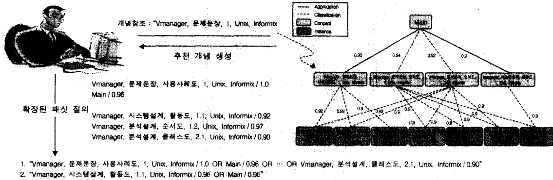
(그림 2) 확장된 패킷 질의 구성 과정
