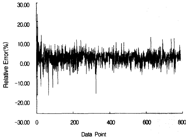
(그림 14) \ln(FP) 이용 \ln(\frac{E}{FP^6}) 추정모델 상대오차
