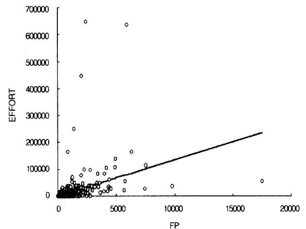
(그림 2) E와 FP 관계 선형회귀
