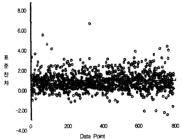
(그림 12) \ln\left(\frac{E}{FP^6}\right) vs. \ln(FP) 관계 모델 표준잔차
