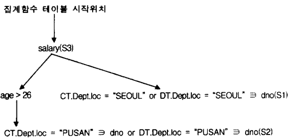
(그림 11) 집계함수 처리 구조
