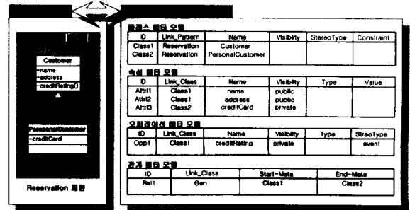
(그림 5) 패턴 메타정보의 데이터베이스 구축
