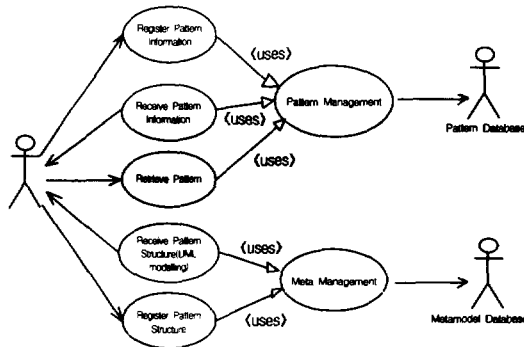
(그림 2) 검색 시스템의 유스케이스 다이어그램
