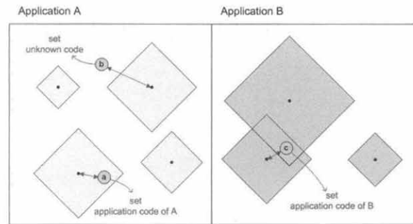
(그림 1) 통계 시그니처 기반 트래픽 분류의 예시
