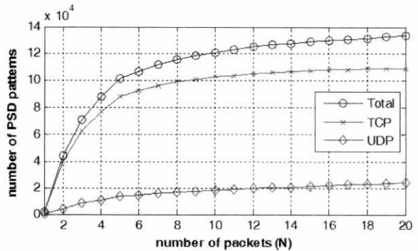
(그림 3) 데이터 패킷 수에 따른 PSD 패턴의 양
