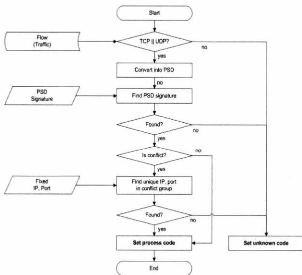
(그림 8) 트래픽 분류 알고리즘의 순서도
