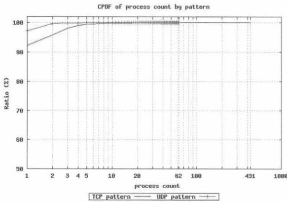
(그림 5) 충돌 프로세스 수에 따른 PSD 패턴 비율
