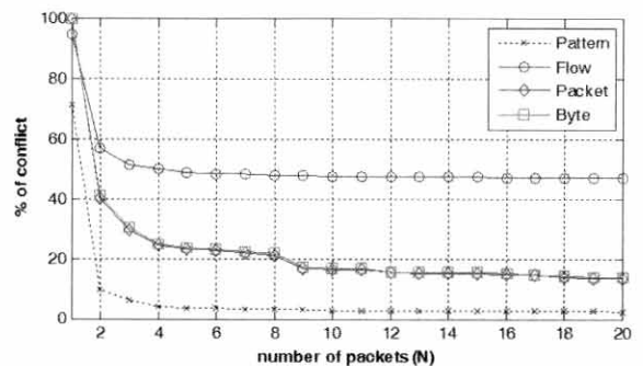
(그림 4) 데이터 패킷 수에 따른 충돌 트래픽의 양
