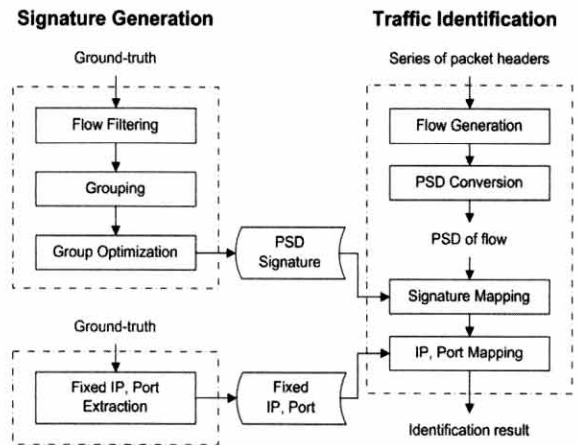
(그림 7) 통계 시그니처 생성과 분류 방법론의 개요
