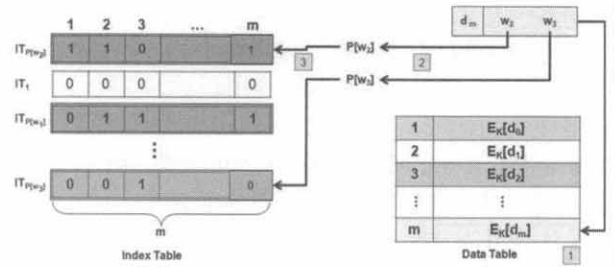
(그림 12) 문서 삽입 과정
