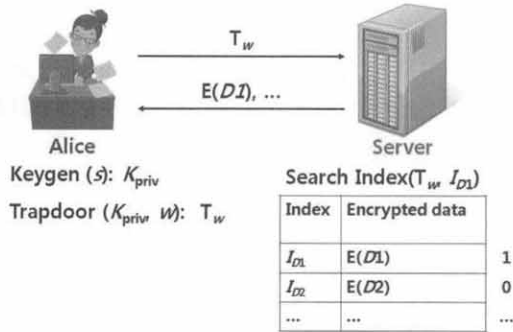
(그림 4) Secure index의 문서 검색 개념도
