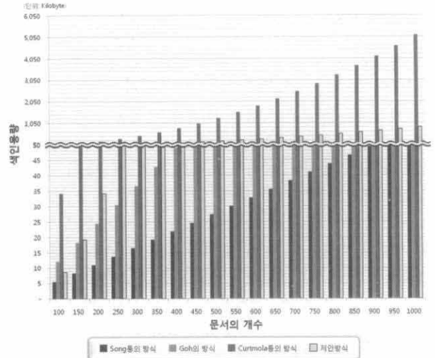
(그림 14) 문서 개수에 따른 색인용량 비교
