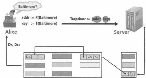
(그림 6) SSE의 검색 과정
