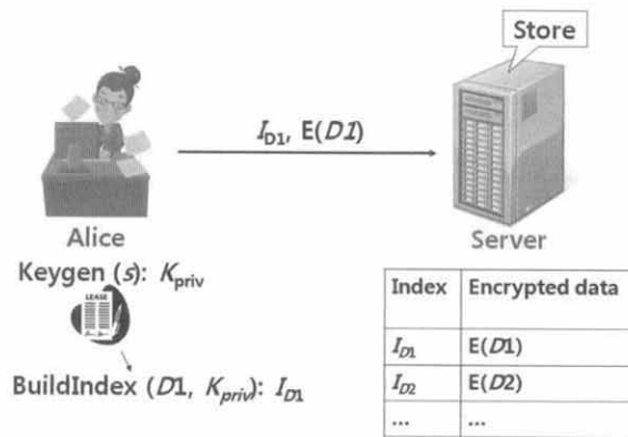
(그림 3) Secure index의 색인 생성 개념도
