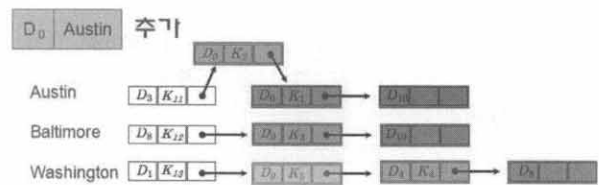
(그림 7) SSE 문서 추가 방법
