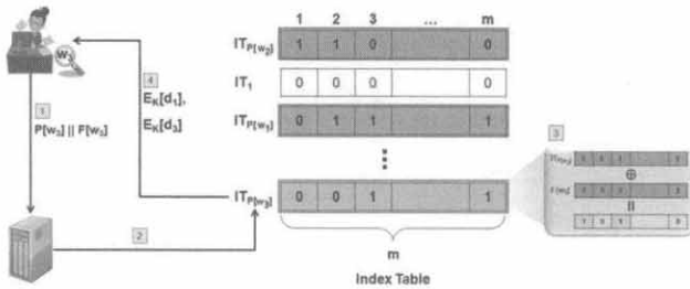
(그림 11) 문서 검색 과정
