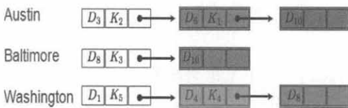
(그림 5) SSE 색인 구조
