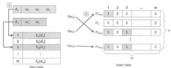
(그림 9) 각 테이블에 문서 정보 추가
