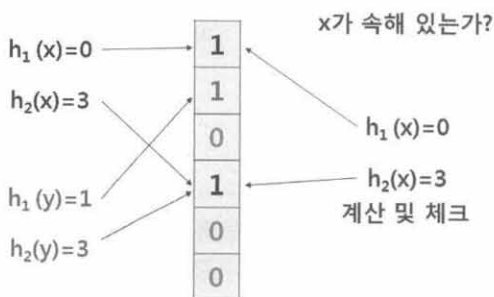
(그림 2) Bloom filter 예시
