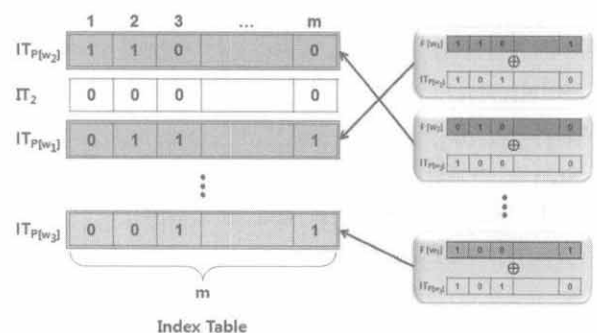
(그림 10) 색인 테이블에 마스킹 수행
