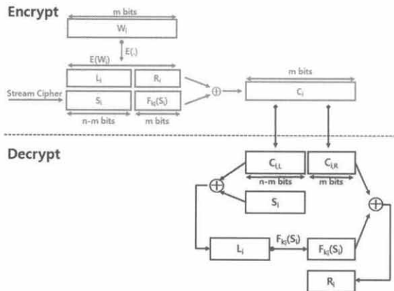
(그림 1) Song et al. 방식의 키워드 암호/복호화 과정
