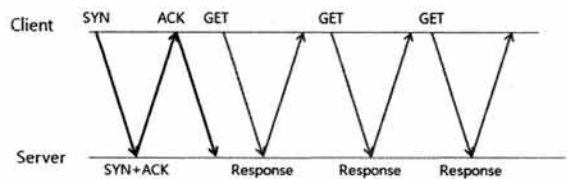
(그림 2) 단일 TCP connection 안에 다중 GET Request
