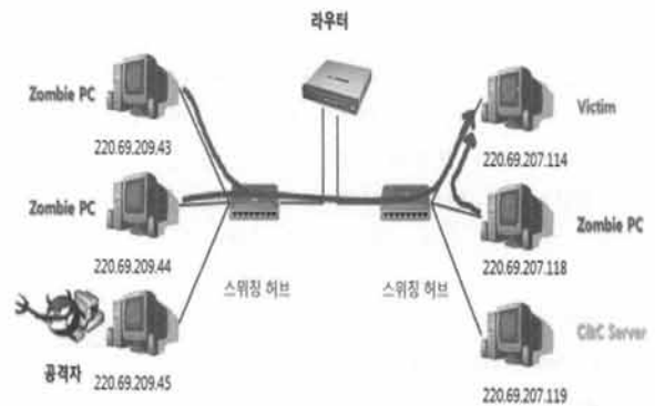
(그림 14) 공격 패킷 로그 수집 네트워크 환경
