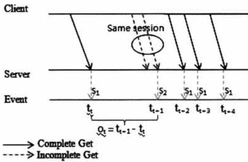
(그림 6) ALAB S1, S2 상태 정의
