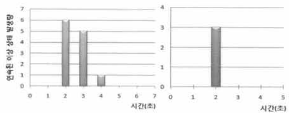
(a) C1 관련 S2 발생량 (b) C2 관련 S2 발생량 (그림 10) 정상 패킷에서 발생한 S2 발생 샘플
