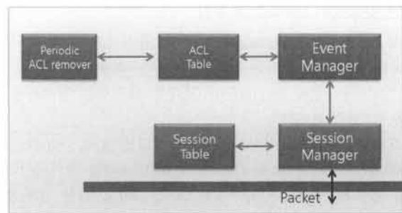
(그림 5) ALAB 탐지 시스템 구성도
