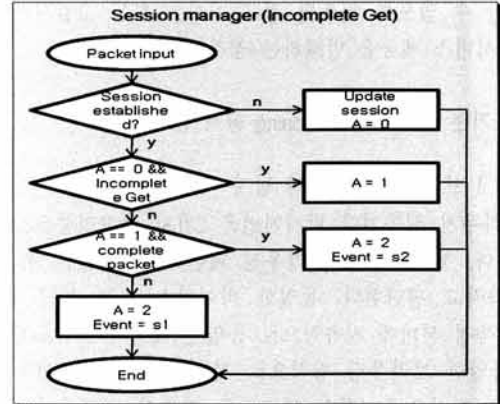
(그림 7) Session manager incomplete GET 탐지 알고리즘
