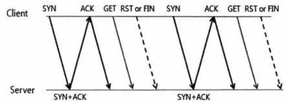
(그림 1) HTTP GET Request 공격 패킷 흐름
