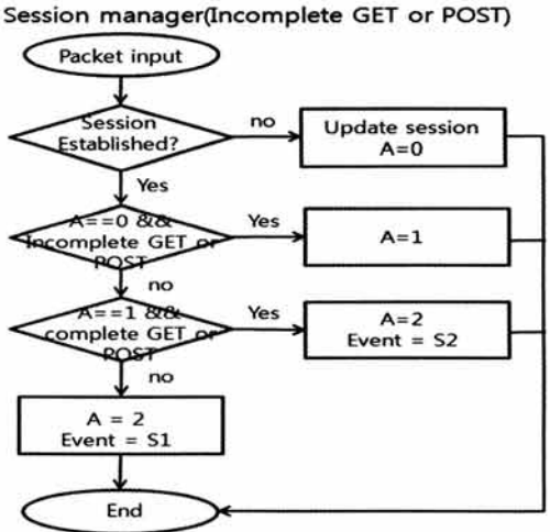
(그림 9) 확장된 Session manager incomplete GET 탐지 알고리즘
