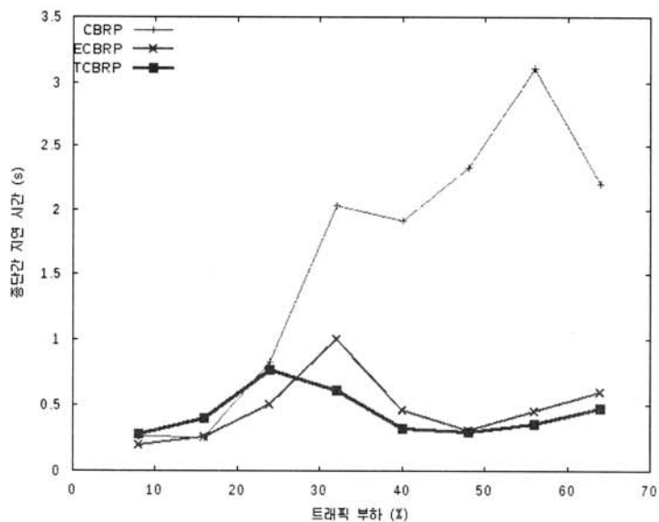
(그림 6) 불균일 네트워크에서의 전송 지연 시간 비교
