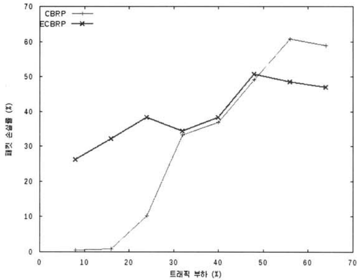
(그림 2) 불균일 분포 네트워크에서의 패킷 손실률
