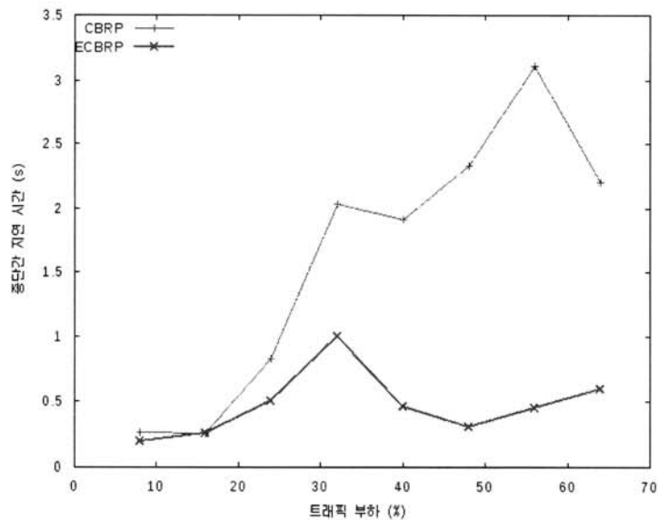
(그림 3) 불균일 분포 네트워크에서의 전송 지연 시간
