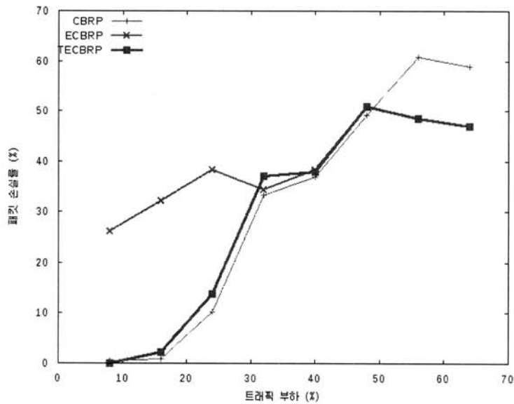
(그림 5) 불균일 네트워크에서의 패킷 손실률 비교
