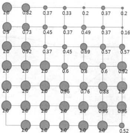
(그림 10) LGR 노드별 수신율(5 Joule)
