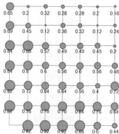
(그림 9) LIGR 노드별 수신율(1 Joule)
