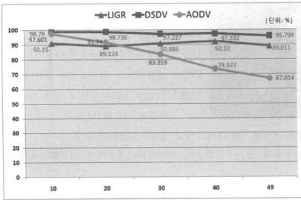
(그림 28) 평균 잔여 에너지(1.0sec)
