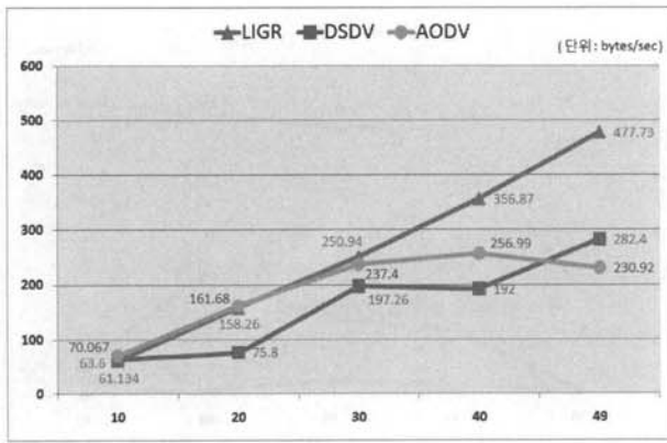
(그림 22) 네트워크 처리율(1.0sec)
