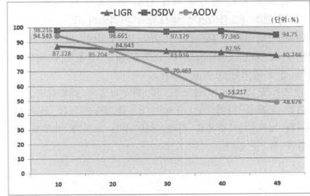
(그림 27) 평균 잔여 에너지(0.5sec)
