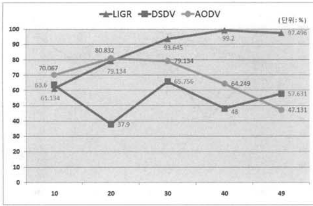
(그림 16) 평균 수신율(1.0sec)
