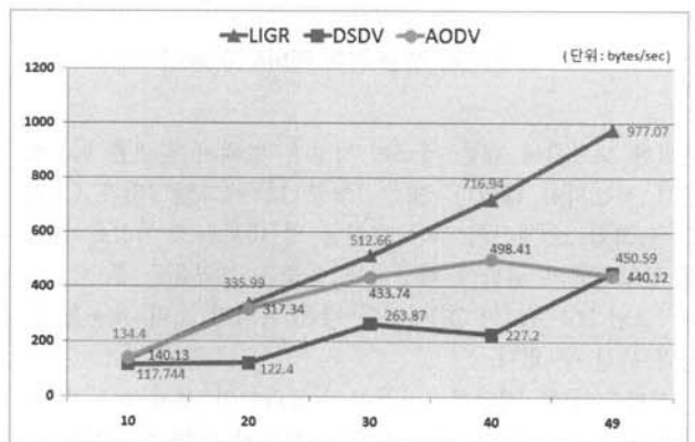
(그림 21) 네트워크 처리율(0.5sec)
