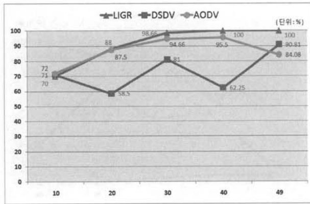
(그림 24) 네트워크 참여율(0.5sec)
