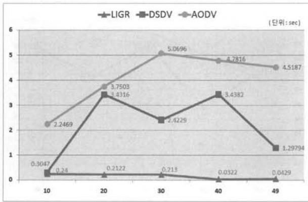
(그림 18) 평균 지연 시간(0.5sec)
