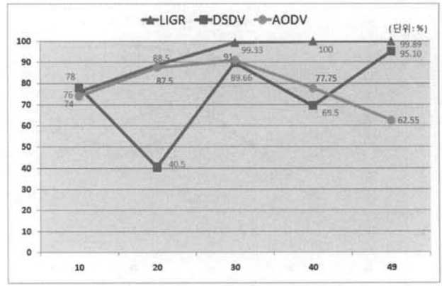
(그림 23) 네트워크 참여율(0.3sec)
