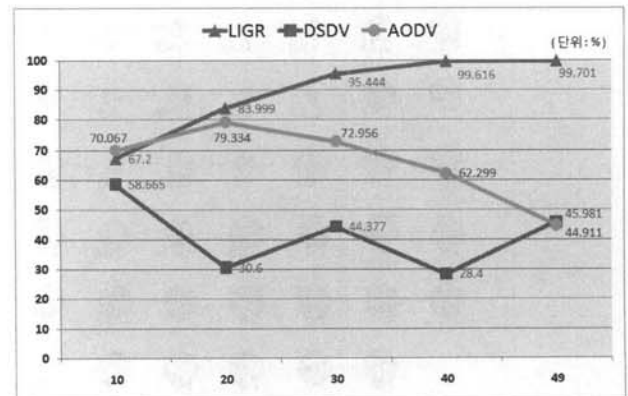
(그림 15) 평균 수신율(0.5sec)
