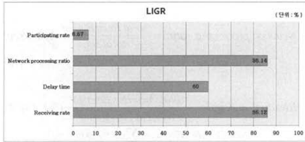
(그림 12) 7×7 환경에서 LGR 대비 LIGR의 성능 향상율(1 Joule)
