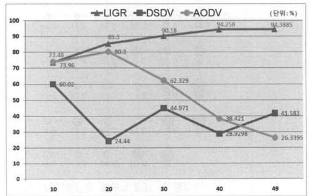
(그림 14) 평균 수신율(0.3sec)
