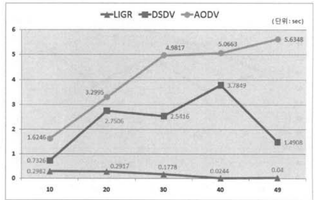
(그림 19) 평균 지연 시간(1.0sec)
