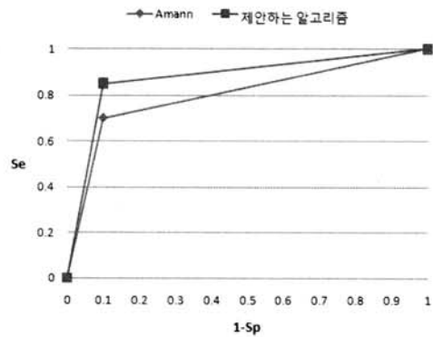
(그림 11) Amann 알고리즘과 제안하는 알고리즘의 ROC 곡선비교
