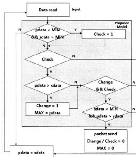
(그림 8) 맥박 측정 알고리즘
