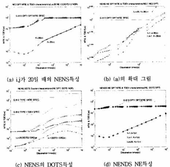
(그림 4) NENS, NENDS SPT상태의 노드클럭특성
