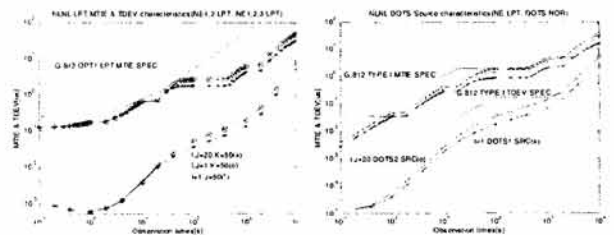
(a) NLNL의 노드 특성 (b) NLNL의 DOTS 특성
