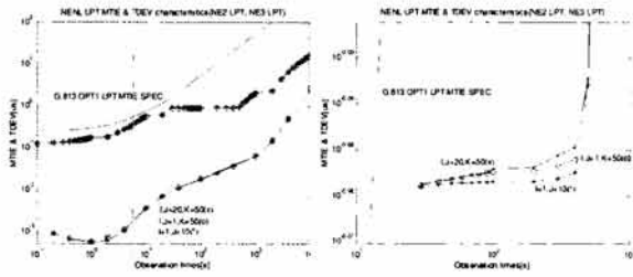
(a) NENL의 노드 특성 (b) (a)의 확대 그림
