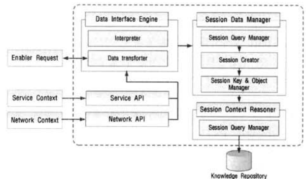
(그림 4) 제안하는 세션 제어 기법의 구조
