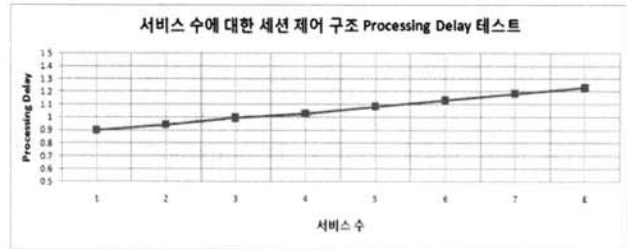
(그림 8) 서비스 수에 대한 세션 제어 처리 시간
