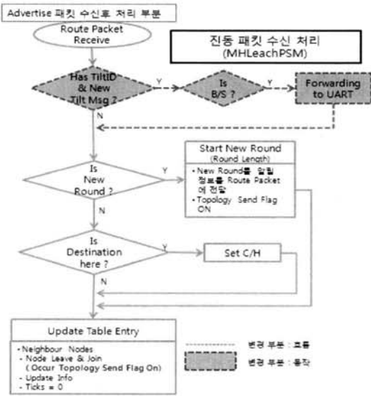
(그림 14) 충격 센서를 활용한 Leave & Join 처리부
