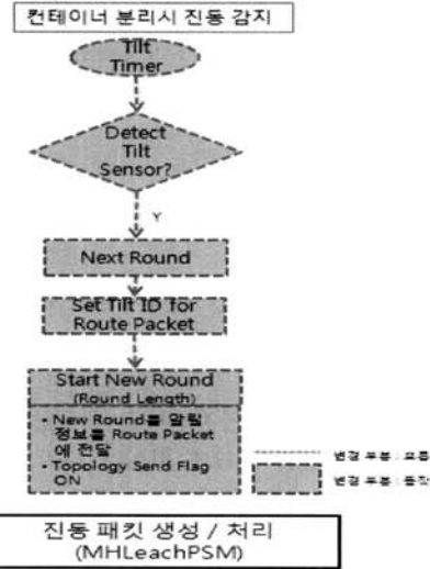
(그림 15) 진동 패킷의 생성 및 처리에 관한 플로우차트
